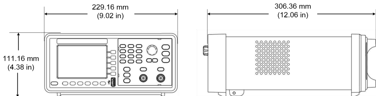
Рис. 1. Размеры прибора
